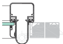
KFI Pfostenprofil
