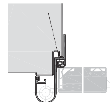
EFI Renovierungs-Eckzarge über bestehender Stahlzarge
