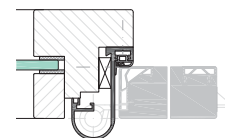
HFI für Kombination mit bauseitigem Holzstock
