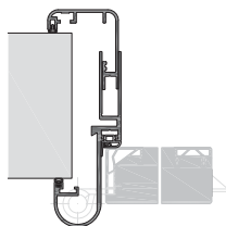
EUROFI Umfassungszarge
