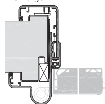
RENOFI Renovierungszarge
